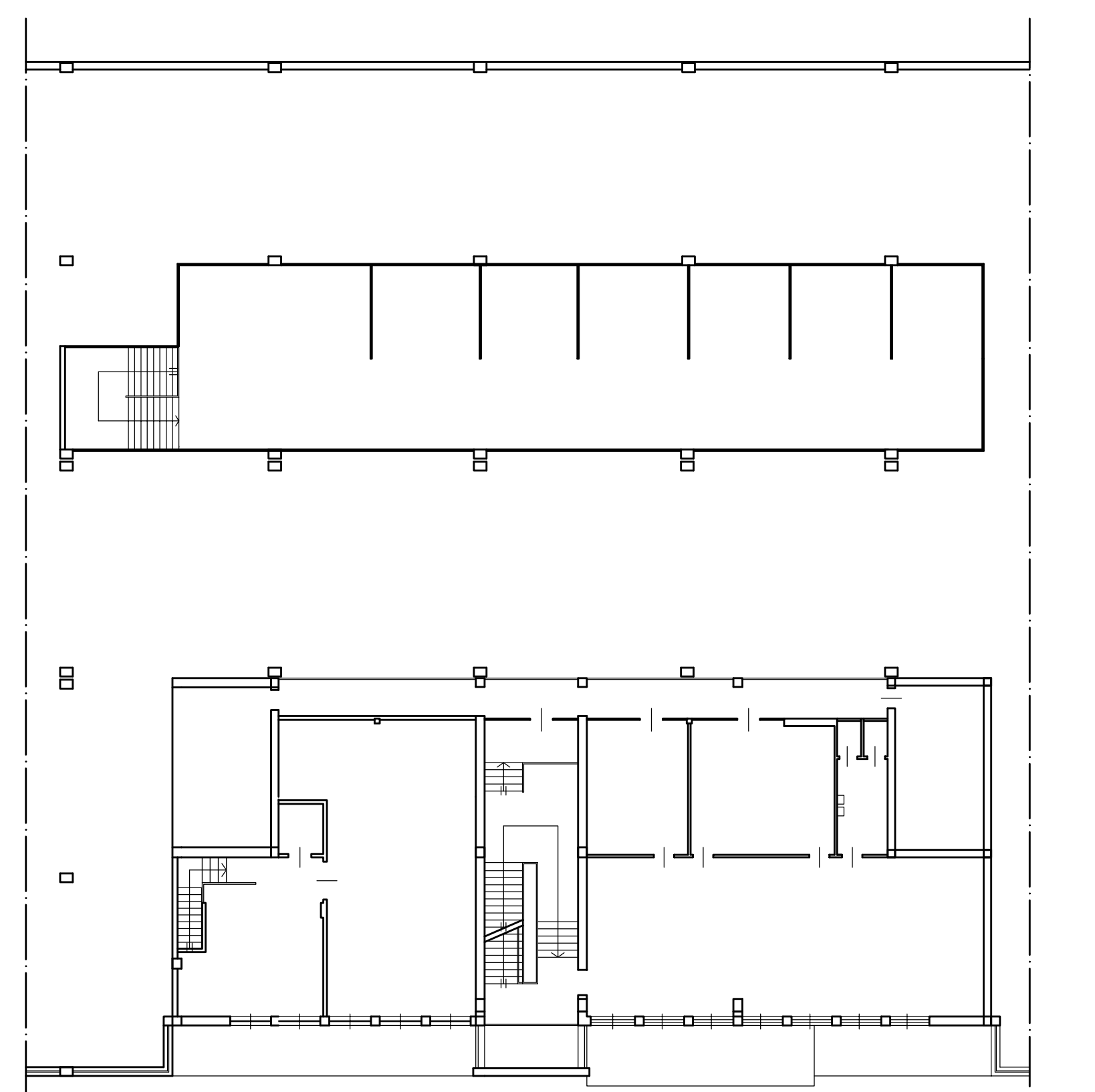
VIA PERUGIA PIANTA PIANO PRIMO LOCALI COMMERCIALI
