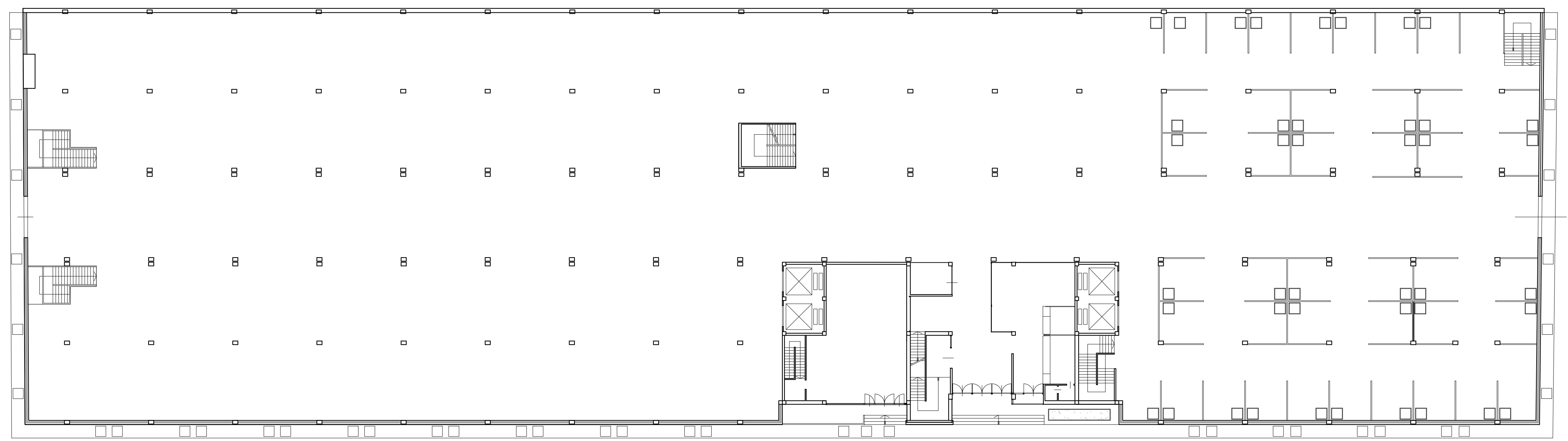
VIA PERUGIA PIANTA PIANO TERRENO LOCALI COMMERCIALI
