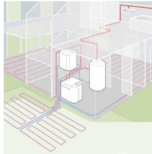
Pompa di calore terra/acqua a sonda orizzontale
