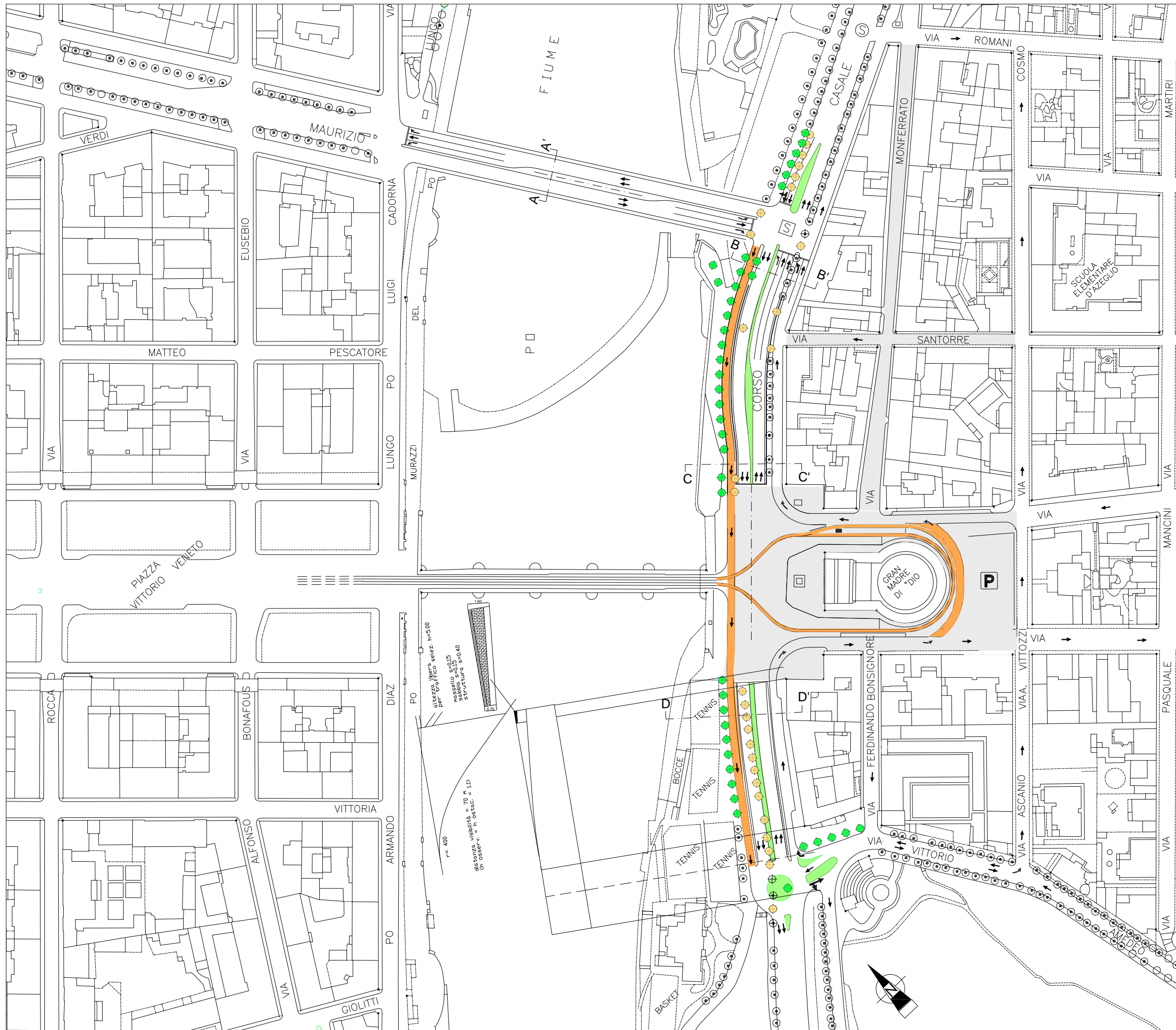
TAV. 11 NODO GRAN MADRE Sottopasso soluzione 2
