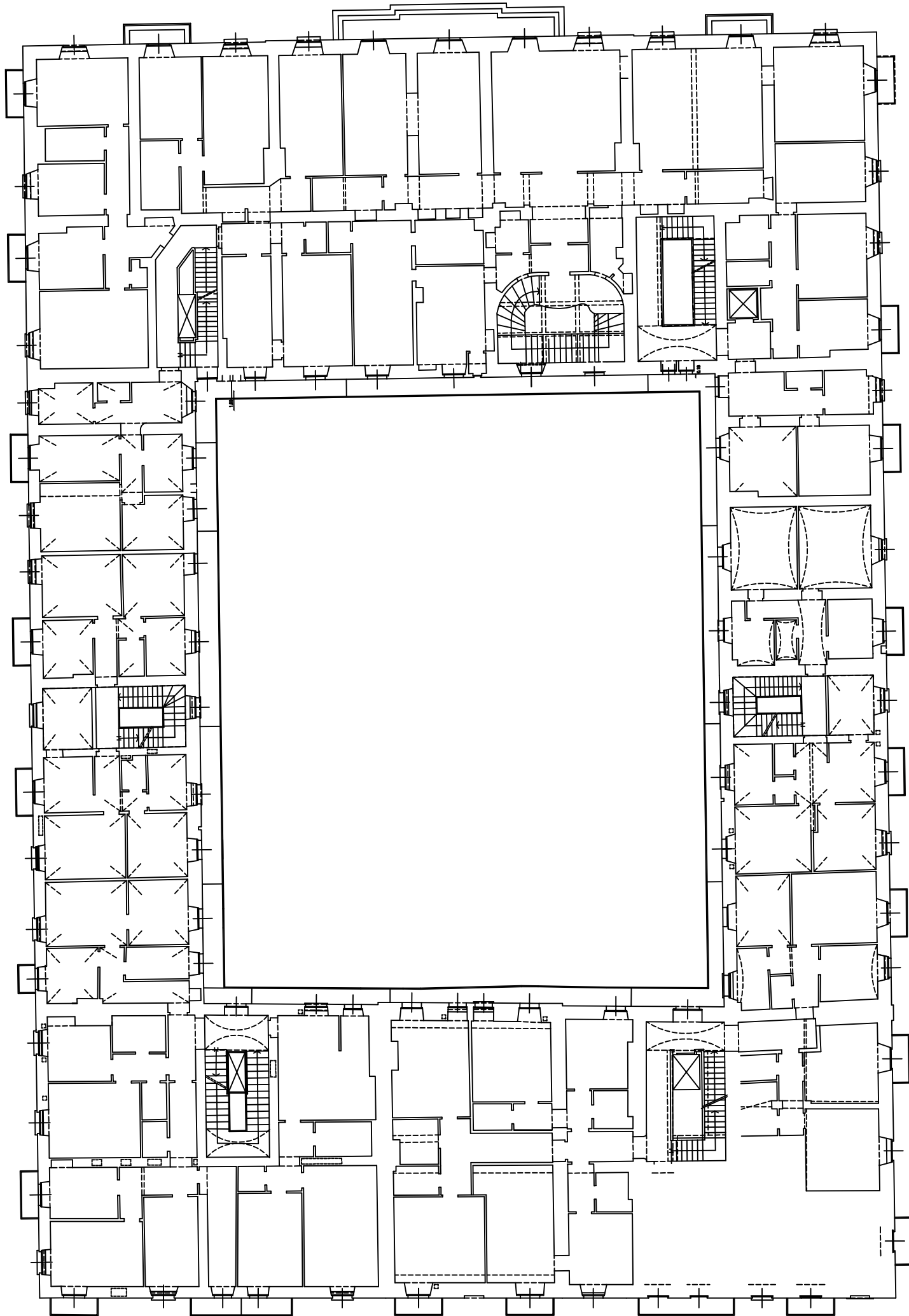
PIANTA PIANO SECONDO
