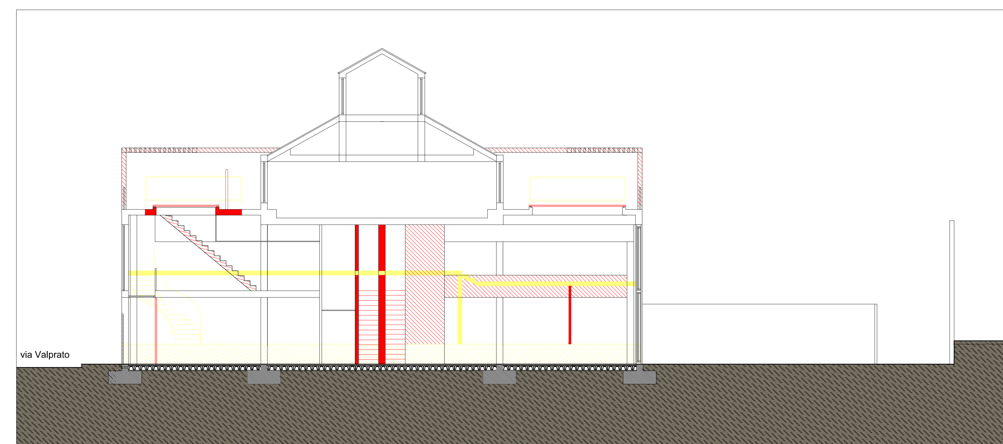
SEZIONE BB
