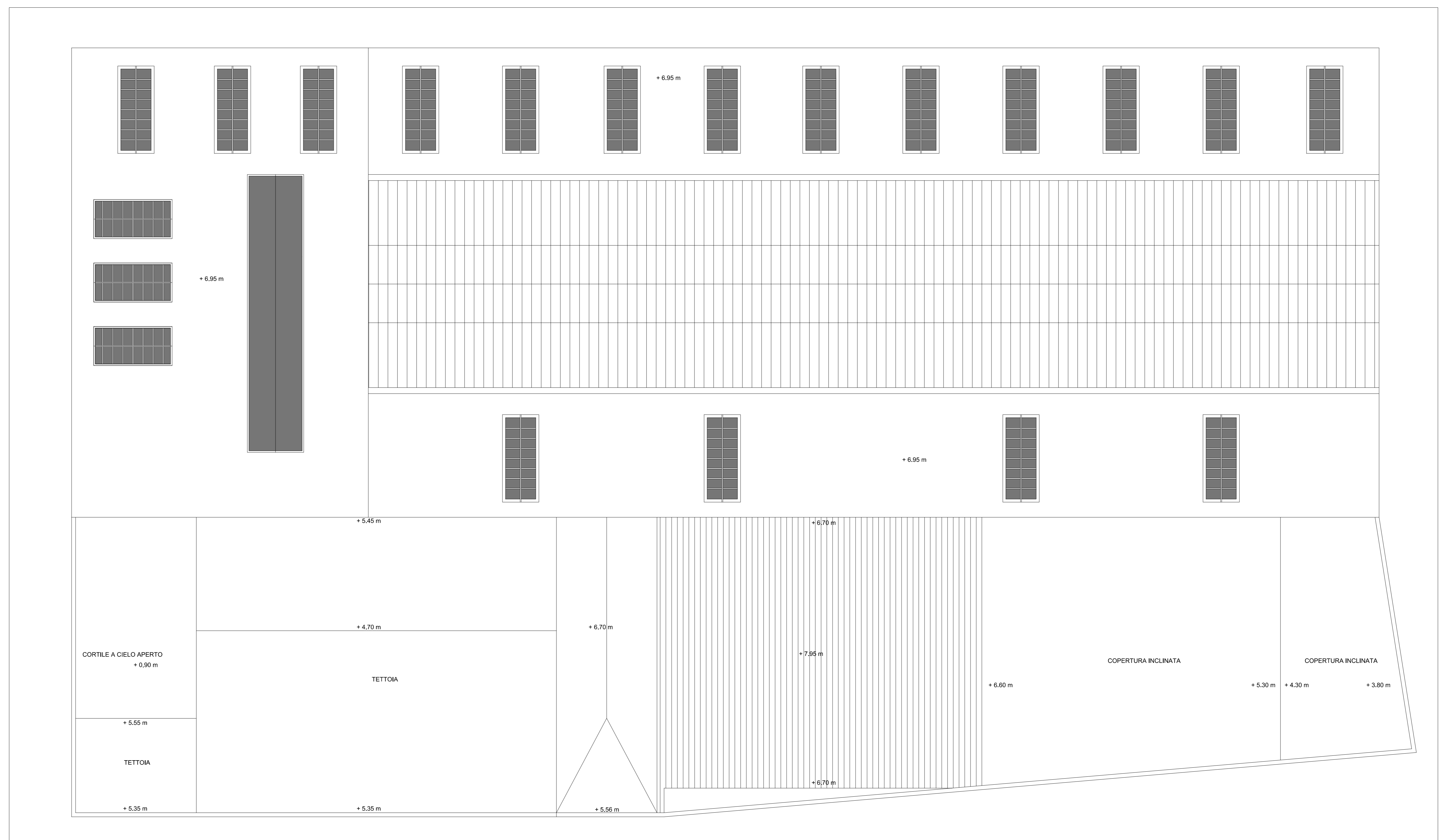
PIANTA COPERTURE
