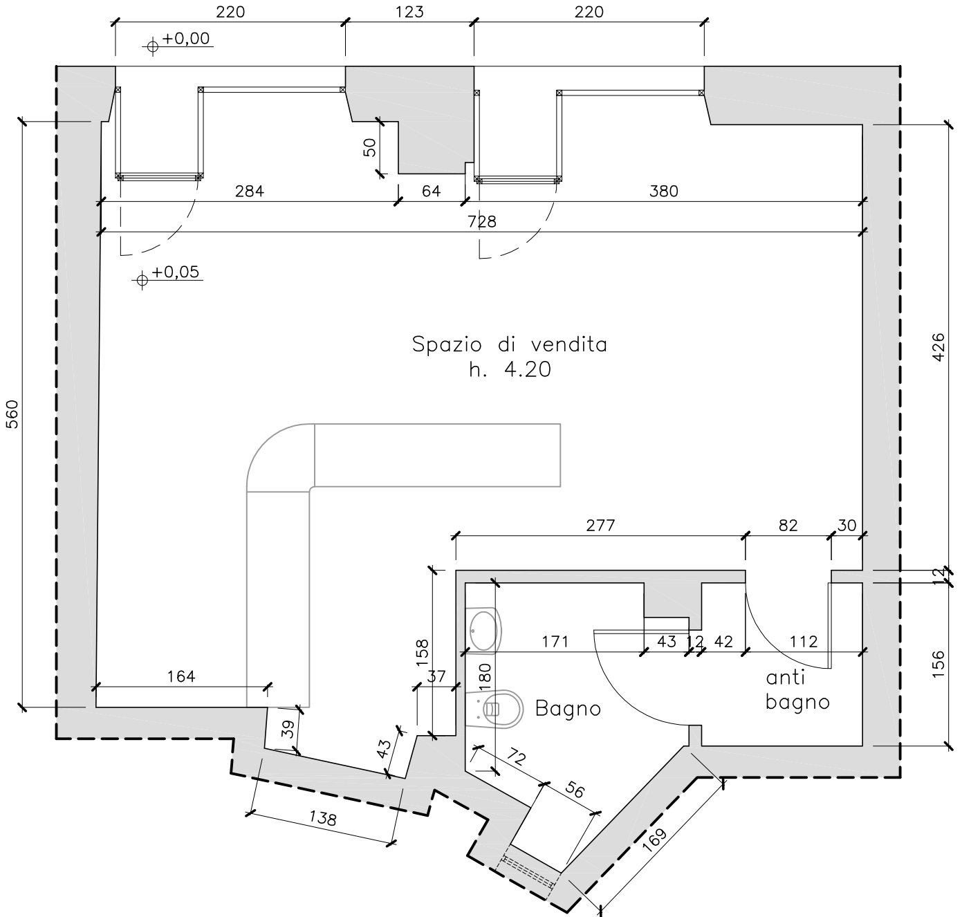
STATO DI PROGETTO scala 1:50
