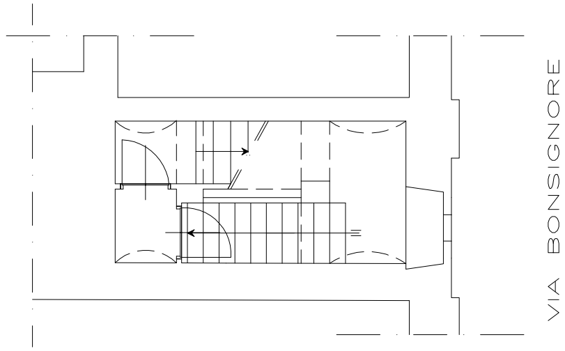
Pianta Piano Interrato
