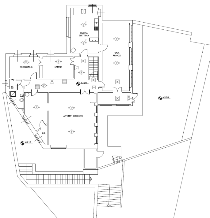
Piano primo
