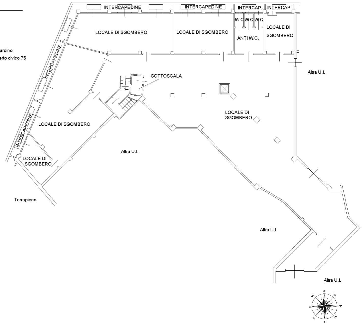
PIANTA PIANO INTERRATO H = 4,12 mt.
