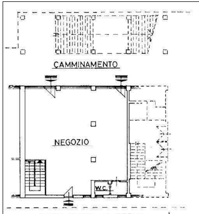
Foglio 1467, p.27, sub. 9 - Stralcio planimetria C.F. - Piano terra - Non in scala
