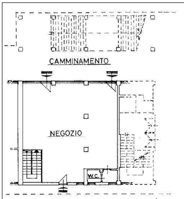
Foglio 1467, p.27, sub. 9 - Stralcio planimetria C.F. - Piano terra - Non in scala
