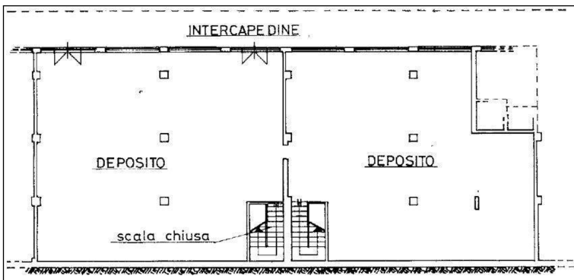
Foglio 1467, p.27, sub. 9 - Stralcio planimetria C.F. - Piano interrato - Non in scala
