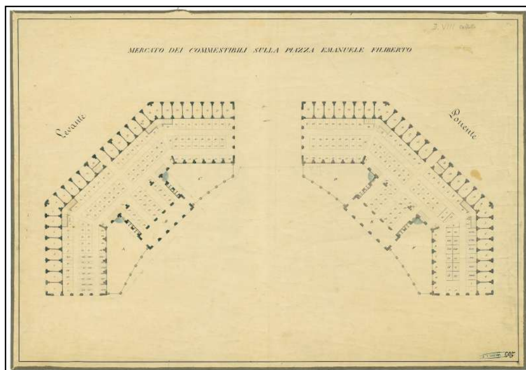
G. Barone, Progetto per padiglioni in muratura, 1836 (ASCT, Tipi e Disegni, 15-22)
