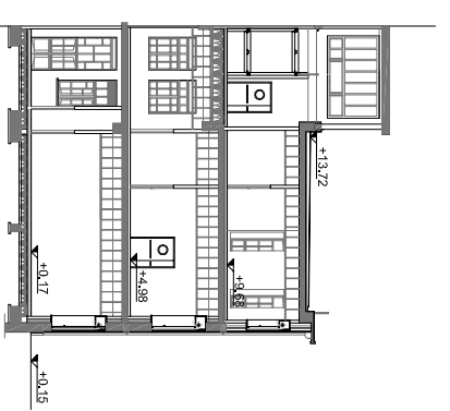
SEZIONE D-D
