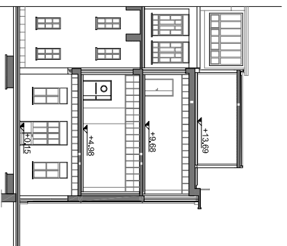
SEZIONE C-C
