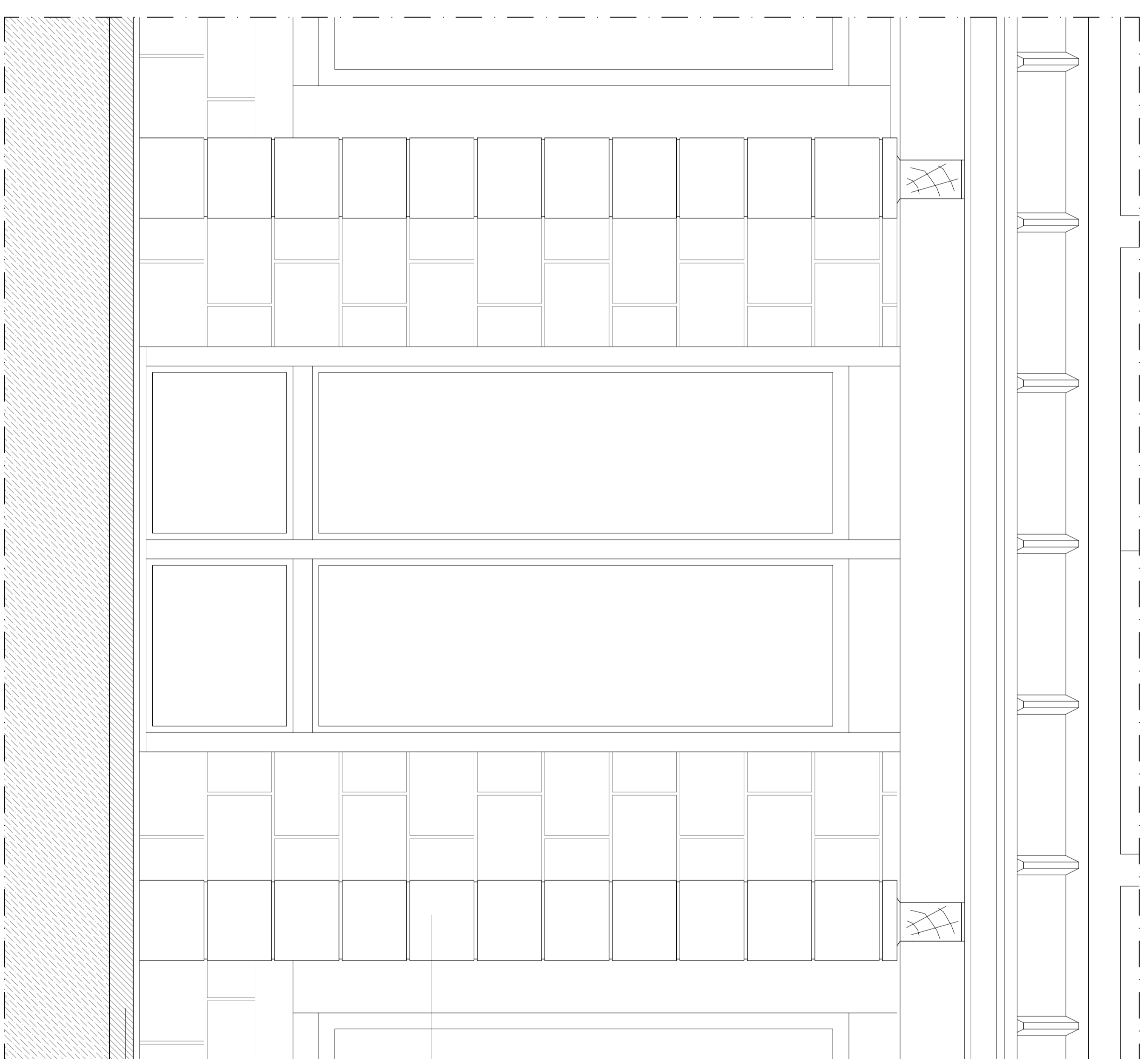
Prospetto passaggio coperto scala 1:10
