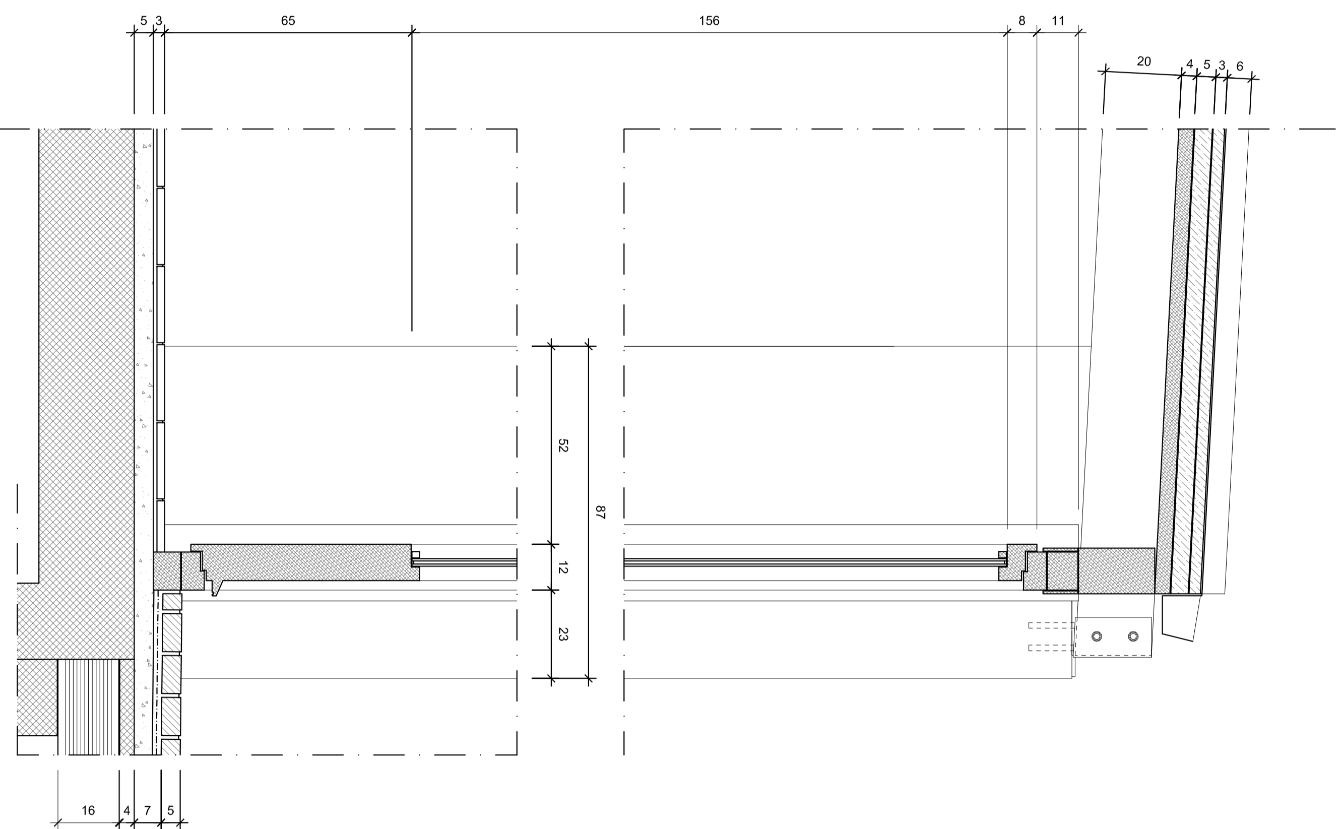
Sezione B-B' scala 1:10
