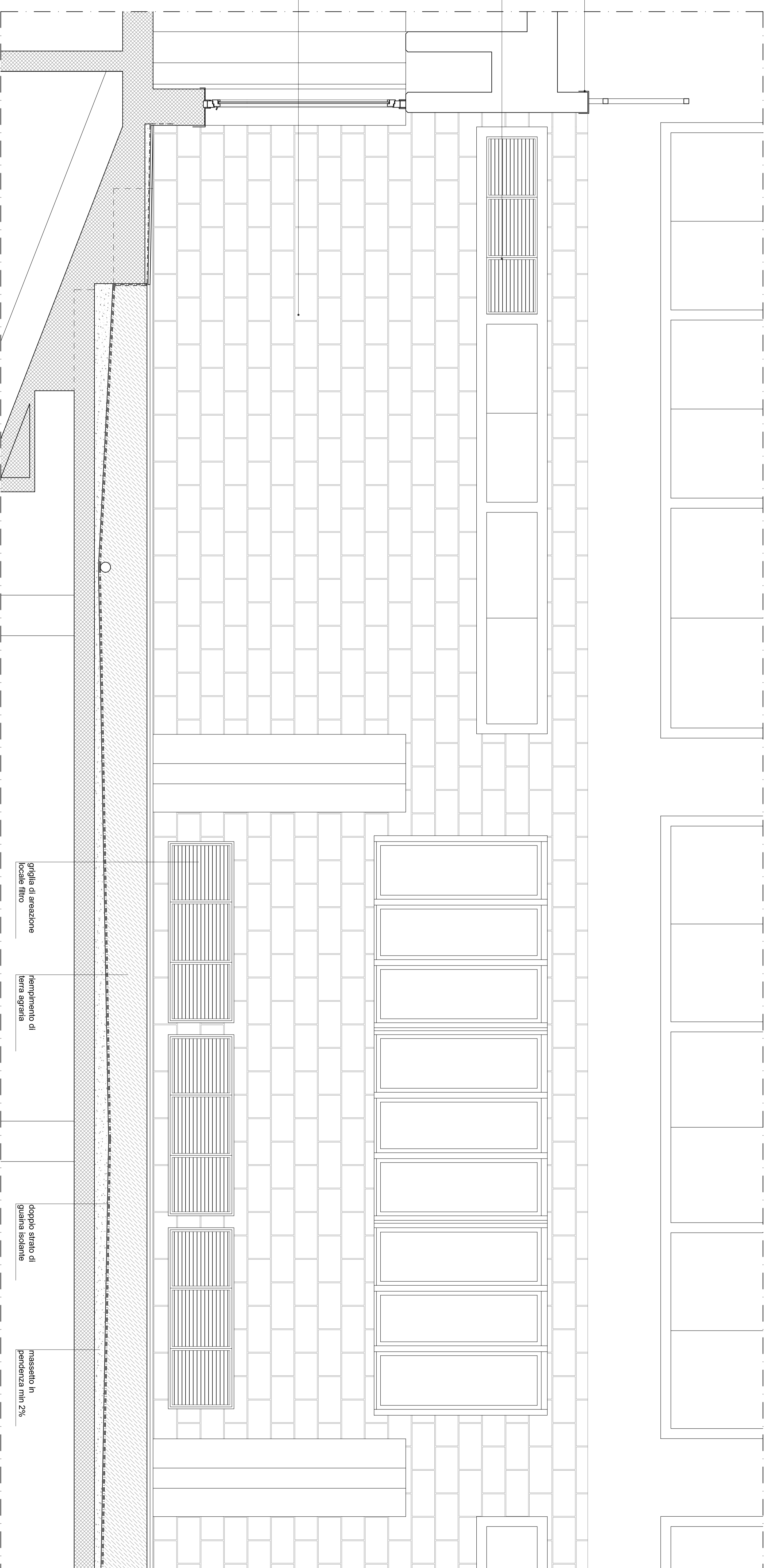
PROSPETTO LATO AILE scala 1:20
